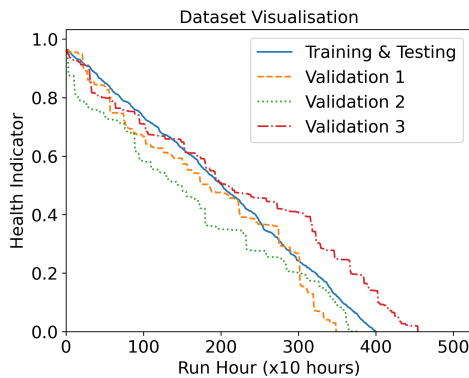
Fig. 3. Dataset Visualisation
