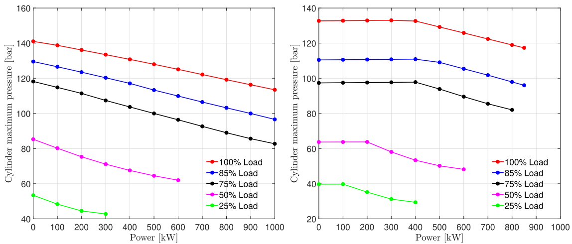
(c) Maximum Cylinder Pressure-Diesel Mode. (d) Maximum Cylinder Pressure-Gas Mode.
