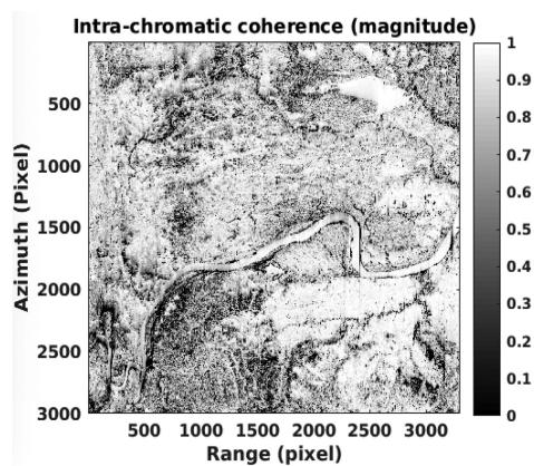
Fig. 20. Infra-chromatic coherence (magnitude).
